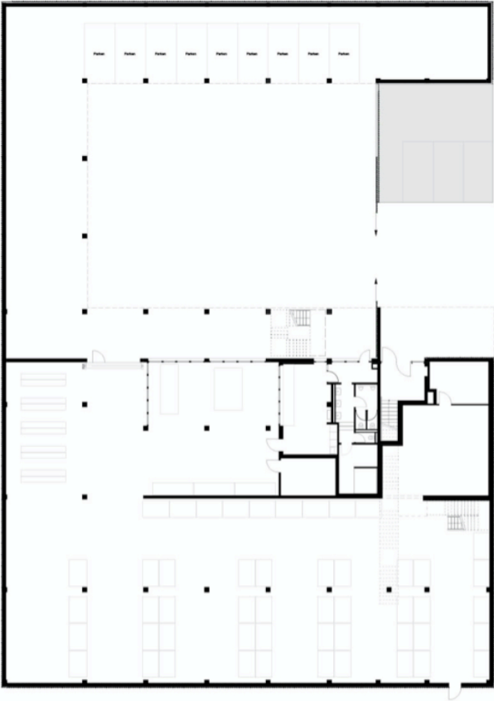
Grundriss EG | Grundriss DG
